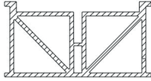
Profil No: 8131 Weight / Ağırlık: 1,110 Kg/m
