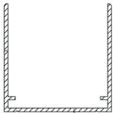
Profil No: 3726 Weight / Ağırlık: 0,545 Kg/m
