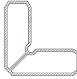
Profil No: 2971 Weight / Ağırlık: 1,442 Kg/m
