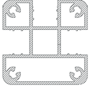
Profil No: 3421 Weight / Ağırlık: 2,512 Kg/m
