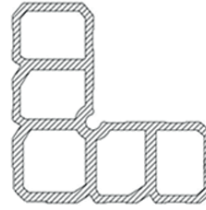
Profil No: 2972 Weight / Ağırlık: 3,440 Kg/m
