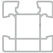
Profil No: 3528 Weight / Ağırlık: 2,992 Kg/m
