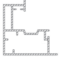
Profil No: 2877 Weight / Ağırlık: 0,726 Kg/m
