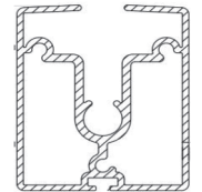
Profil No: 2937 Weight / Ağırlık: 1,201 Kg/m
