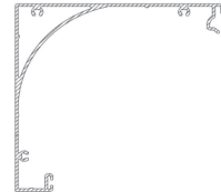
Profil No: 2878 Weight / Ağırlık: 1,585 Kg/m
