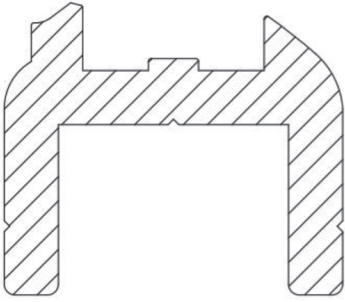
Profil No: 4366 Weight / Ağırlık: 3,875 Kg/m
