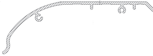
Profil No: 4367 Weight / Ağırlık: 1,767 Kg/m
