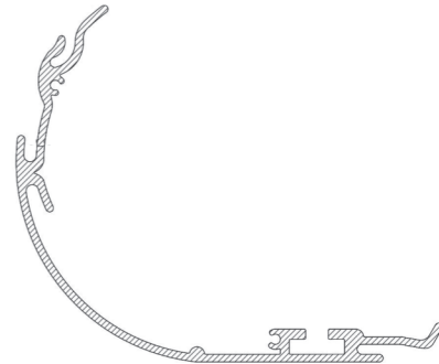
Profil No: 4370 Weight / Ağırlık: 3,512 Kg/m
