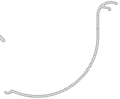
Profil No: 4368 Weight / Ağırlık: 1,035 Kg/m
