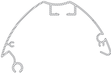
Profil No: 4369 Weight / Ağırlık: 1,735 Kg/m
