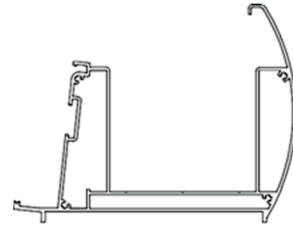
Profil No: 2594 Weight / Ağırlık: 5,619 Kg/m
