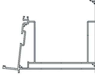
Profil No: 2530 Weight / Ağırlık: 5,399 Kg/m
