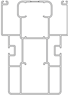
Profil No: 2785 Weight / Ağırlık: 5,084 Kg/m
