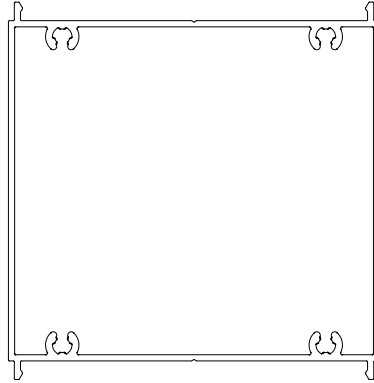
Profil No: 2341 Weight / Ağırlık: 3,028 Kg/m
