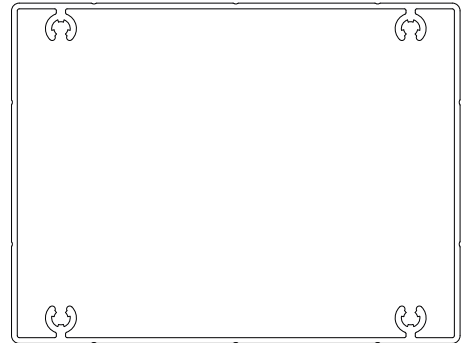
Profil No: 2111 Weight / Ağırlık: 3,044 Kg/m
