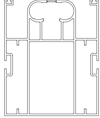
Profil No: 2339 Weight / Ağırlık: 7,827 Kg/m
