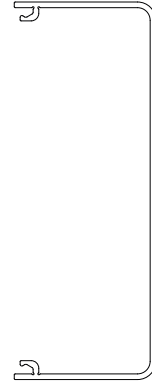
Profil No: 2342 Weight / Ağırlık: 1,055 Kg/m
