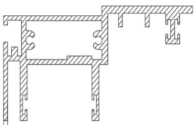
Profil No: 3039 Weight / Ağırlık: 2,110 Kg/m
