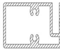
Profil No: 3042 Weight / Ağırlık: 1,210 Kg/m
