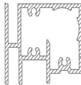
Profil No: 3041 Weight / Ağırlık: 1,450 Kg/m
