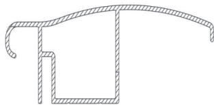
Profil No: 3040 Weight / Ağırlık: 1,572 Kg/m
