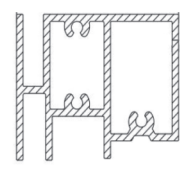
Profil No: 3043 Weight / Ağırlık: 1,390 Kg/m
