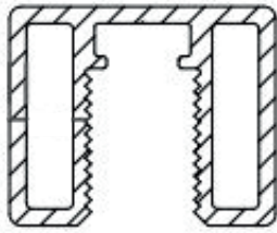
Profil No: 3065 Weight / Ağırlık: 0,370 Kg/m
