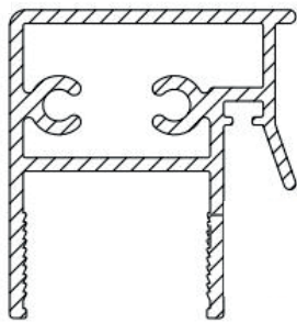
Profil No: 3067 Weight / Ağırlık: 0,800 Kg/m
