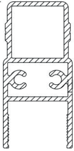
Profil No: 3064 Weight / Ağırlık: 1,030 Kg/m
