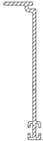
Profil No: 3073 Weight / Ağırlık: 0,540 Kg/m
