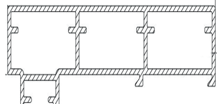
Profil No: 3570 Weight / Ağırlık: 1,772 Kg/m
