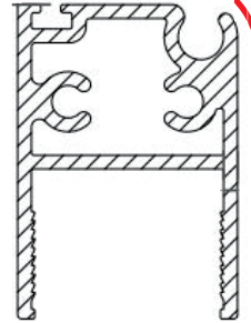
Profil No: 3067 Weight / Ağırlık: 0,800 Kg/m
