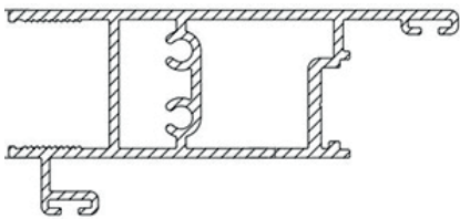
Profil No: 3569 Weight / Ağırlık: 1,257 Kg/m
