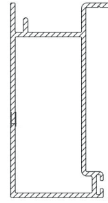
Profil No: 3072 Weight / Ağırlık: 1,170 Kg/m
