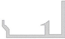
Profil No: 6312 Weight / Ağırlık: 5,596 Kg/m
