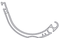
Profil No: 6244 Weight / Ağırlık: 1,645 Kg/m
