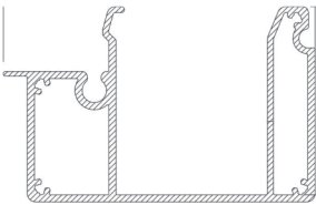
Profil No: 3180 Weight / Ağırlık: 3,905 Kg/m
