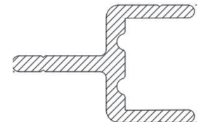
Profil No: 3567 Weight / Ağırlık: 1,390 Kg/m
