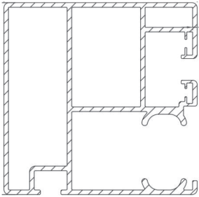
Profil No: 3178 Weight / Ağırlık: 2,981 Kg/m
